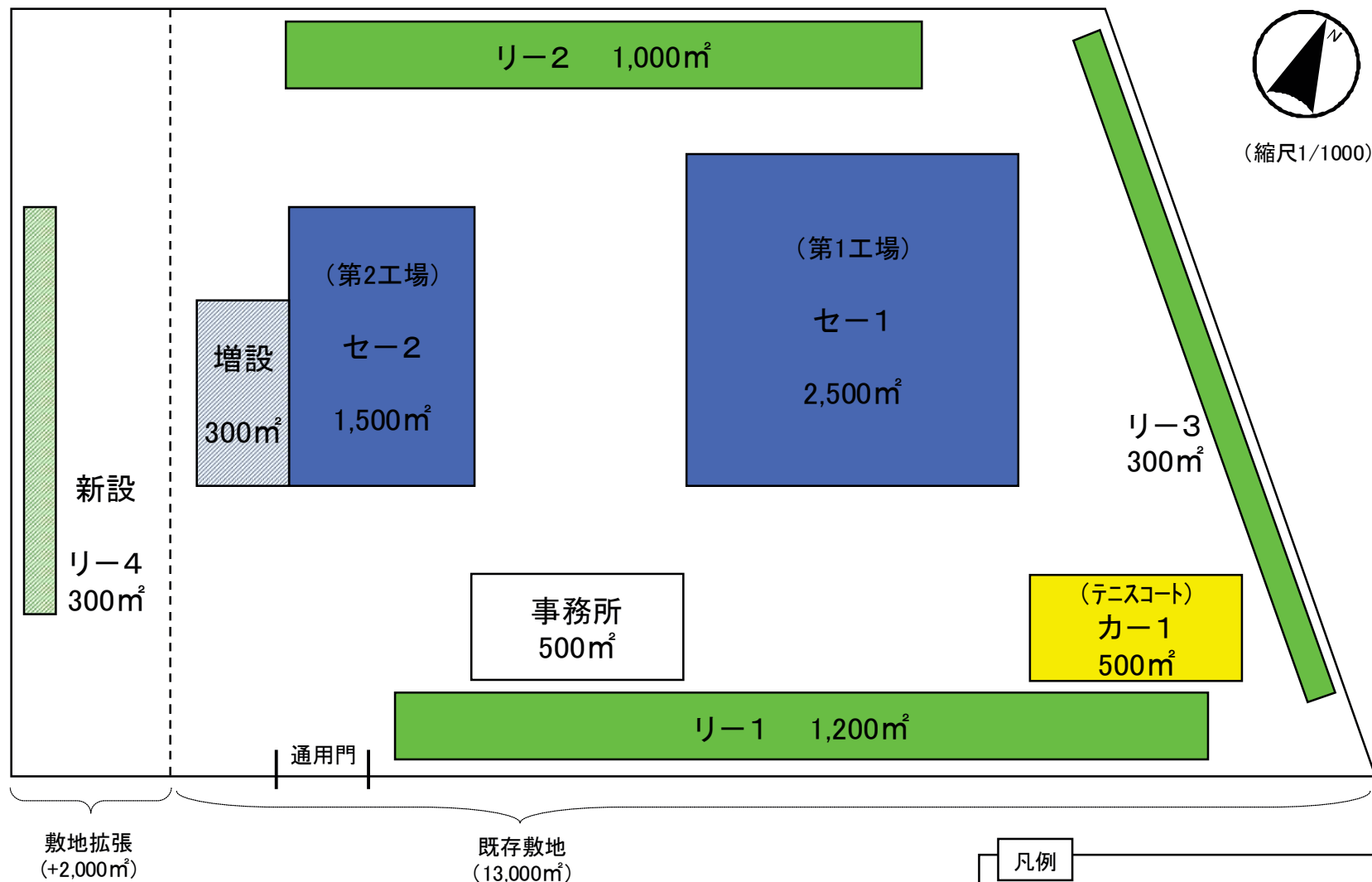
(図1) 生産施設, 緑地, 緑地以外の環境施設その他の主要施設の配置図 (イメージ)
