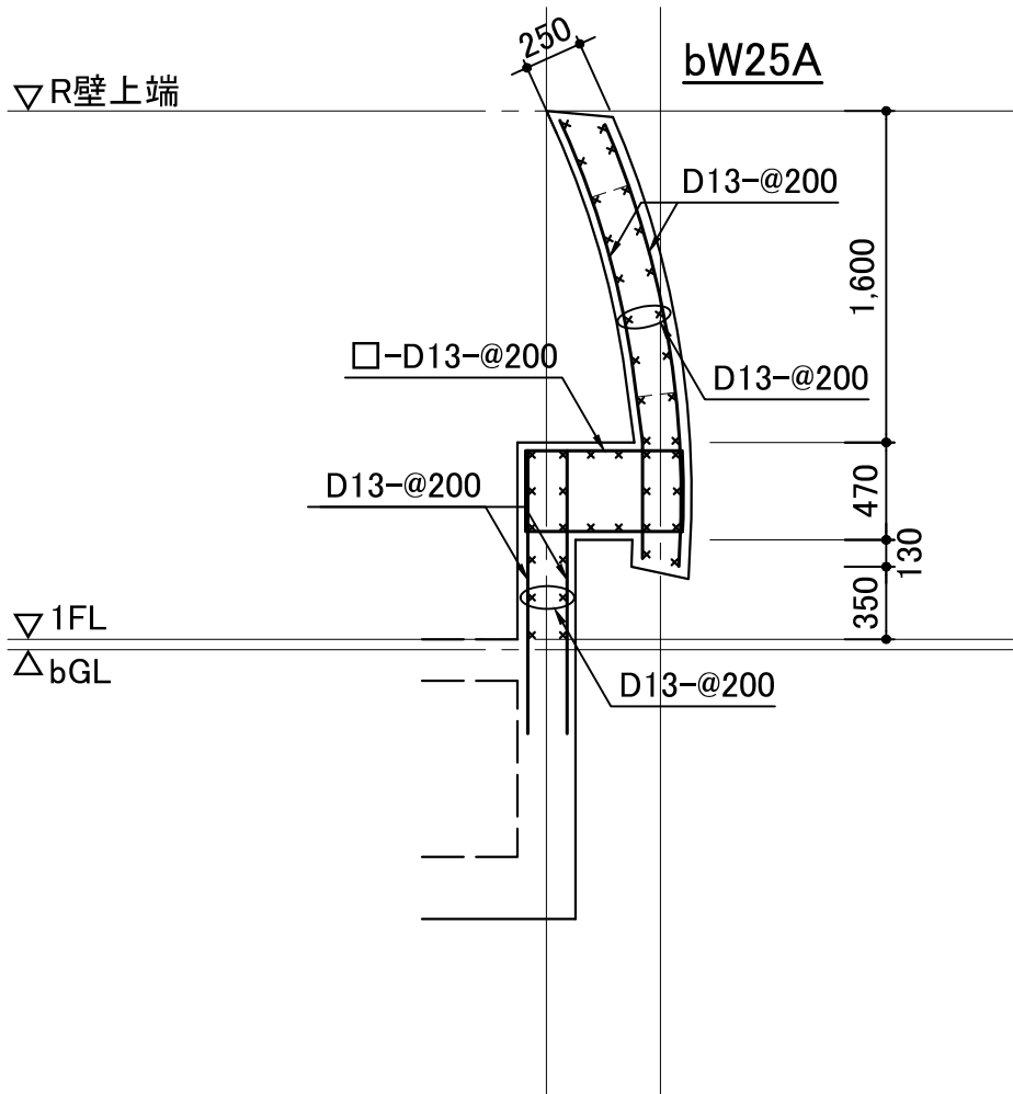
外壁(bW25A)詳細図 1/40 特記なき限り1. 巾止め筋1-D10／m2
