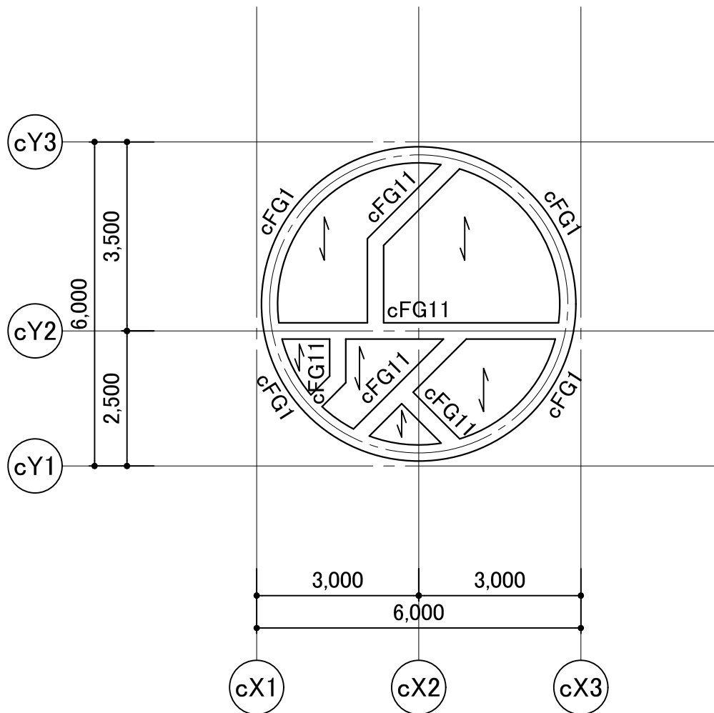
基礎伏図 1/100
