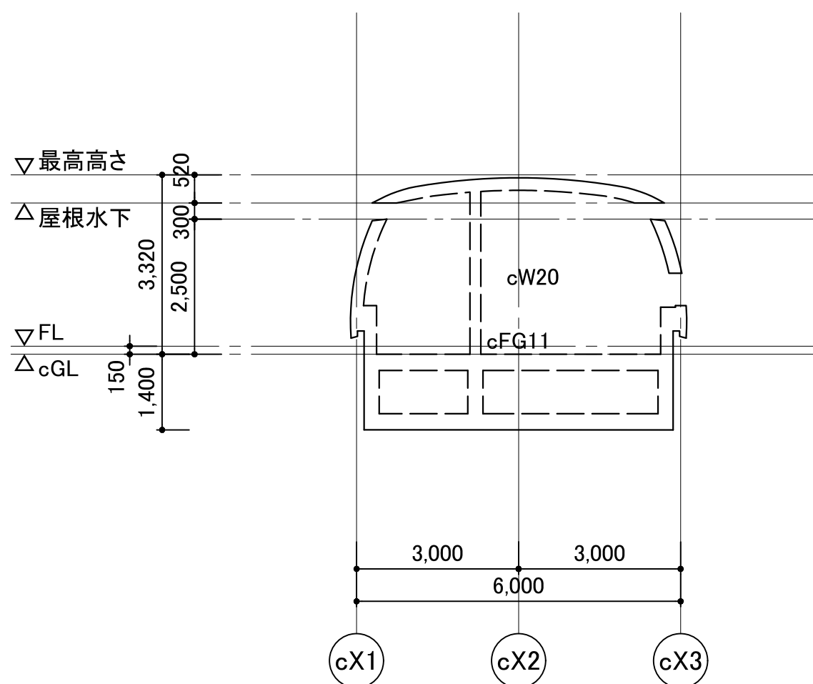
cY2 通 軸組図 1/100
