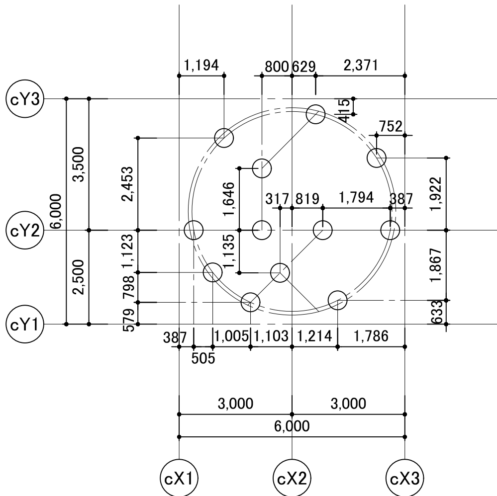
地盤改良伏図 1/100
