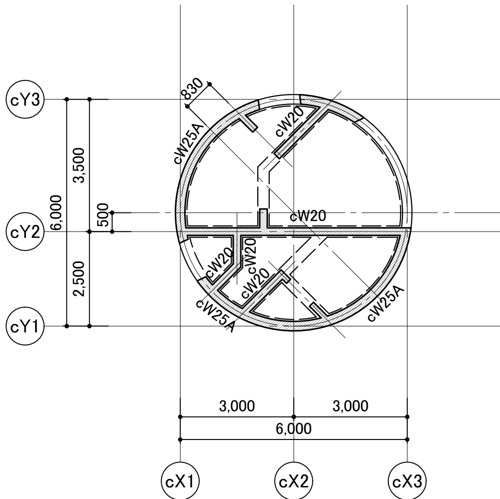
1階伏図 1/100
