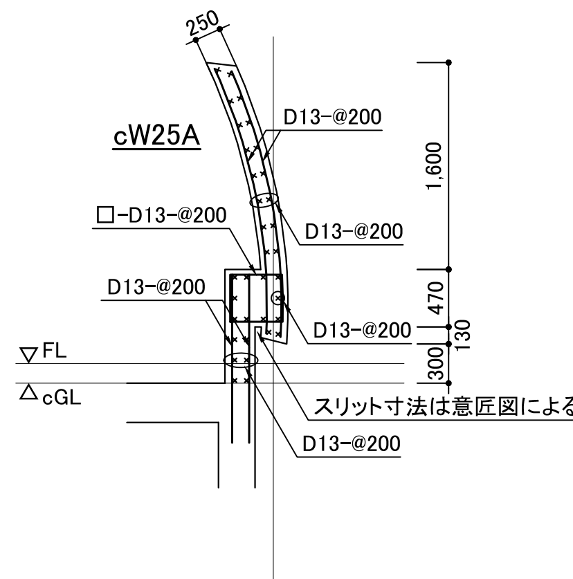
外壁(cW25A)詳細図 1/40 特記なき限り 1. 巾止め筋 1-D10/m2
