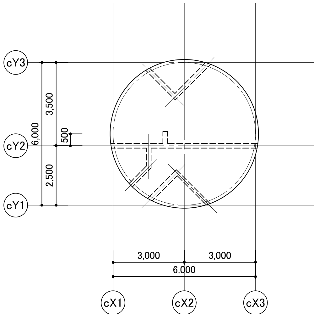
屋根伏図 1/100
