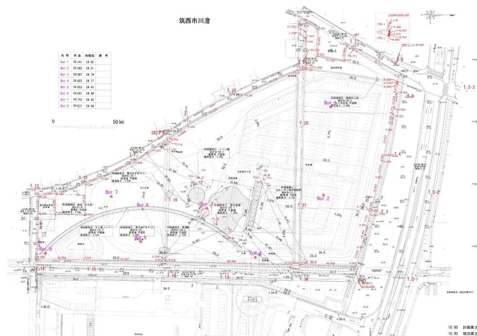
ボーリング位置図
